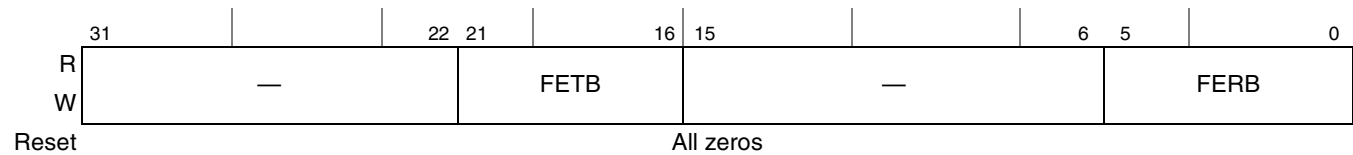
Figure 21-24. Endpoint Flush (ENDPTFLUSH)
