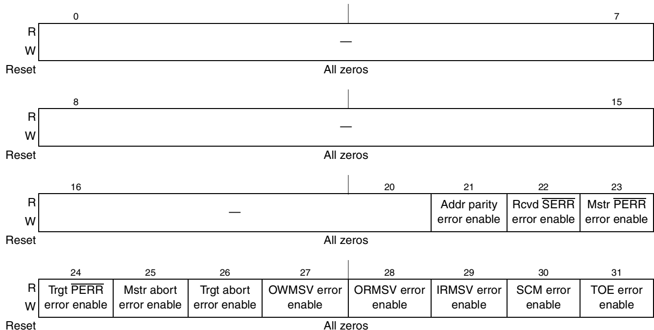
Figure 16-17. PCI Error Enable Register (ERR_EN)
