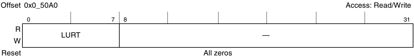
Figure 13-12. UPM Refresh Timer (LURT)
